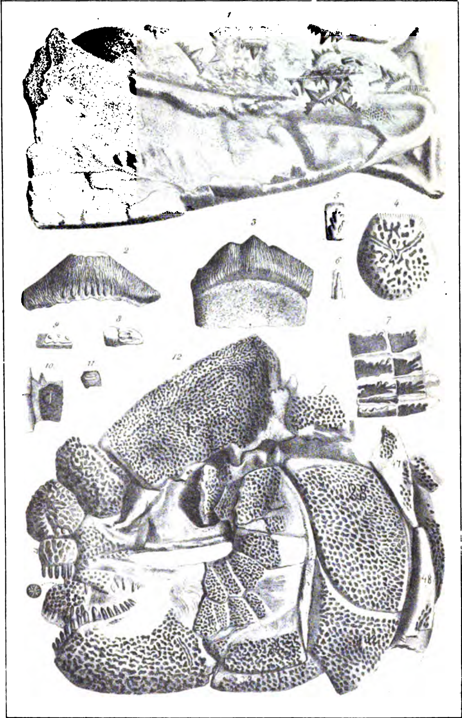
Quenstedt, Jura.
